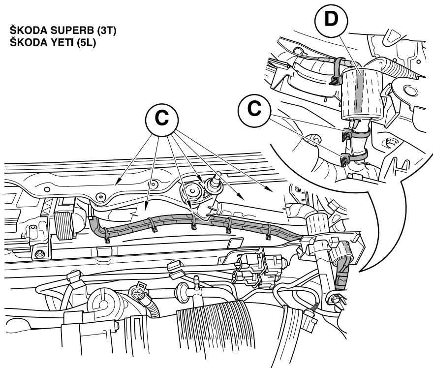
Řídicí jednotka motoru Motorsteuergerät T94a/ viz obr. 4/ siehe Bild 4/ see fig.4 Control unit of the motor
